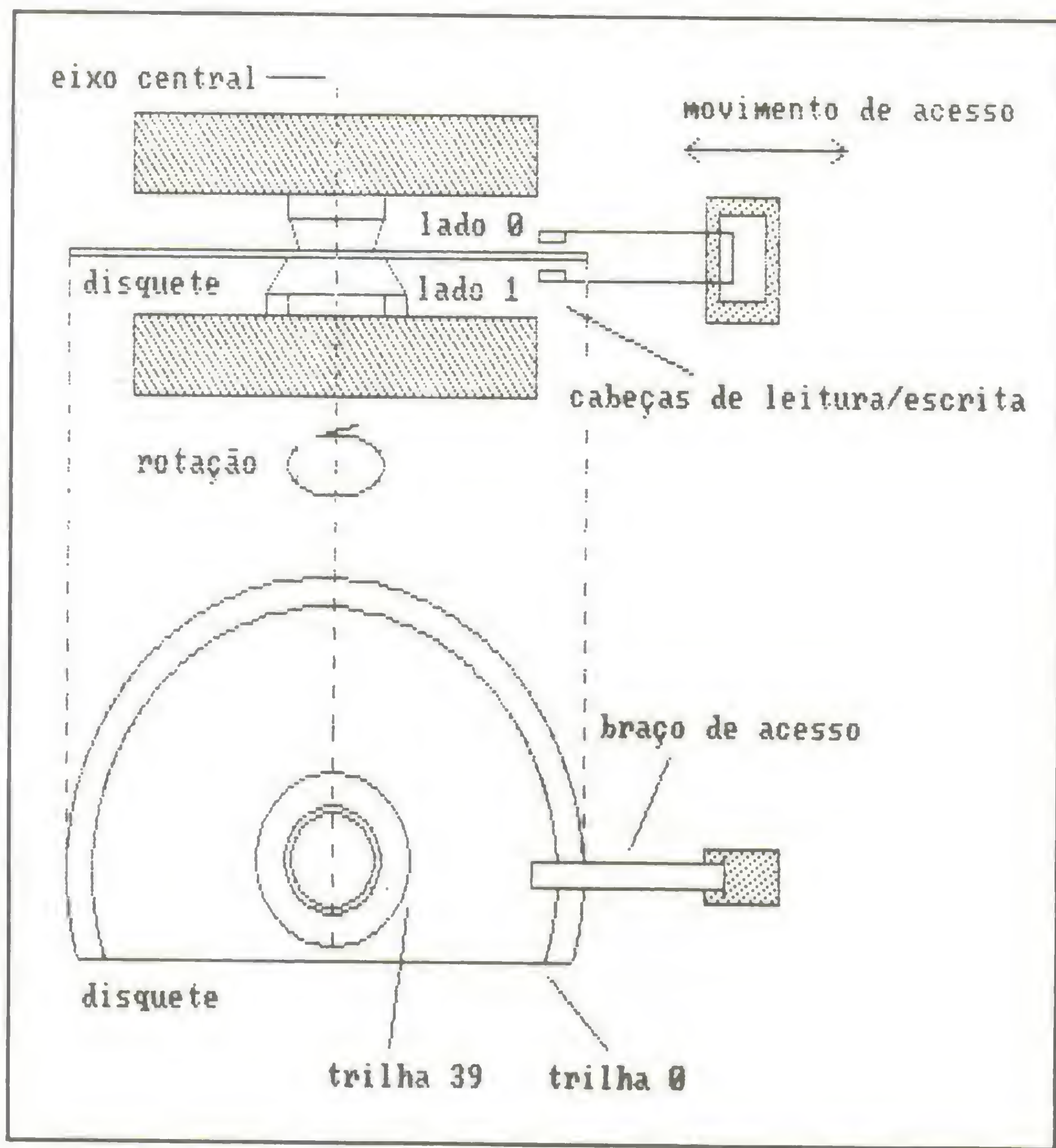
Figura 2: Acionador de disco com um disquete de 5 1/4
